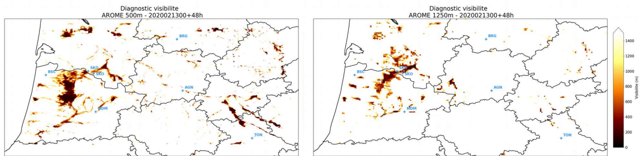
Visibilités prévues par AROME-500m (à gauche) et AROME-1250m (à droite) du 13/02/2020 00h UTC pour le 15/02/2020 00h UTC.
