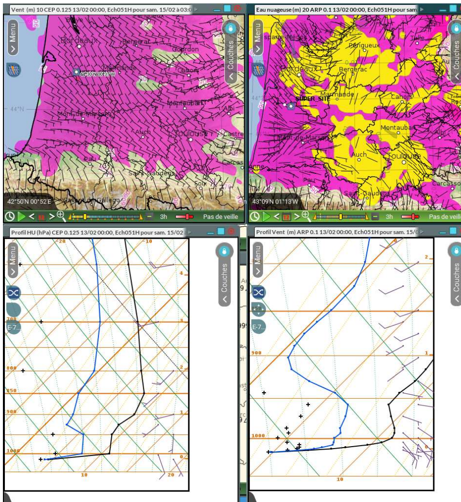
CEP ARPEGE RUN du 12/02/2020 pour le 14/02/2020 03h UTC
