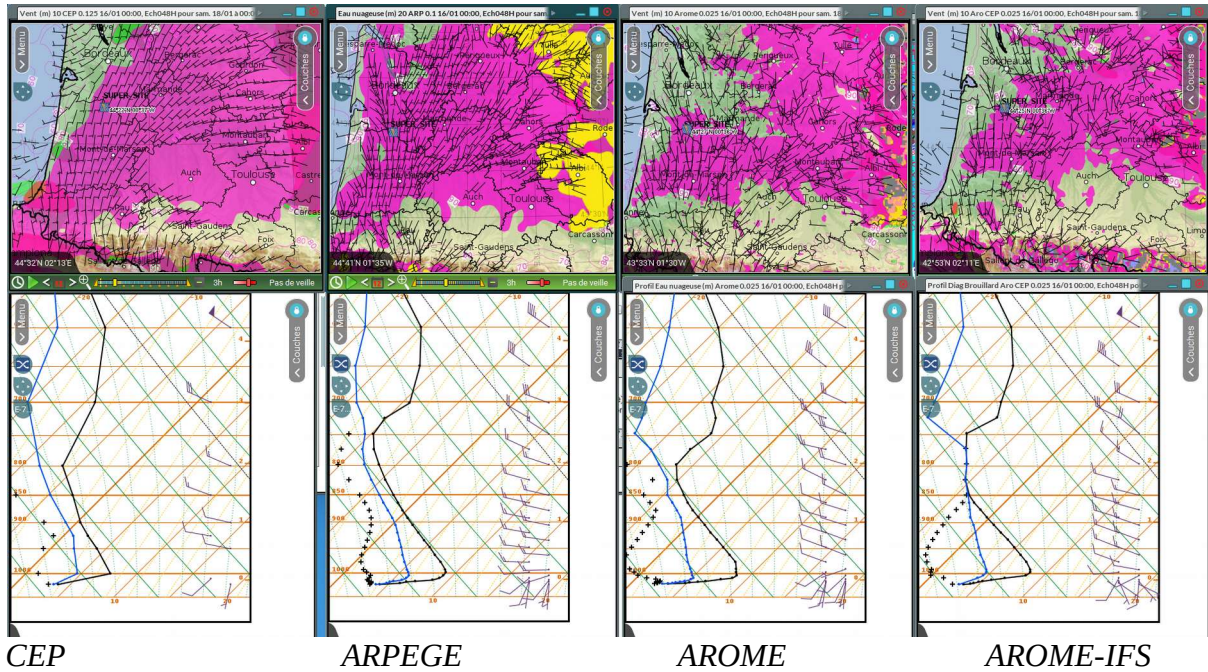
Run 16/01/2020 00UTC pour le 18/01/2020 à 00UTC
