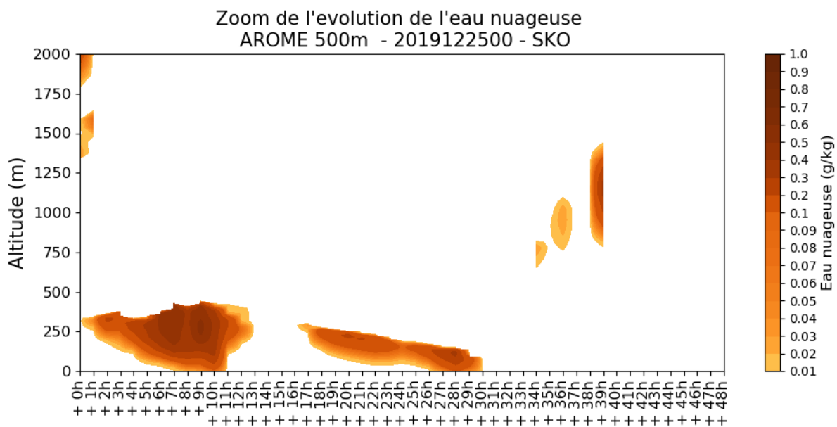
Evolution temporelle sur 48h du contenu en eau nuageuse prévue par AROME 500m Réseau mercredi 25/12 0h
