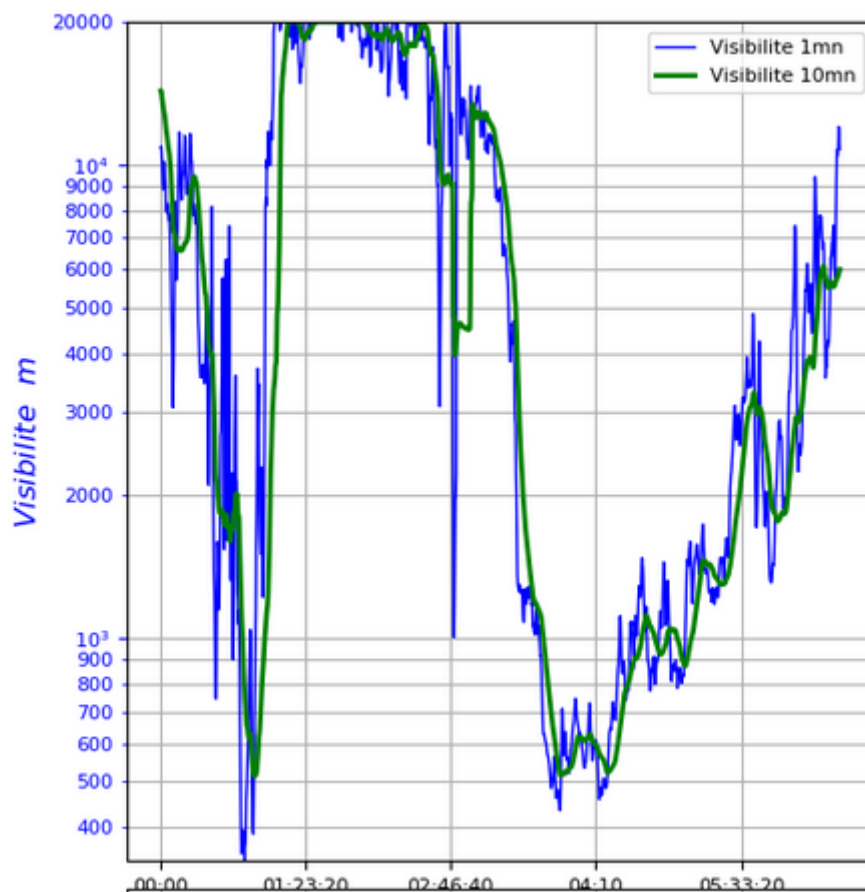
Evolution temporelle de visi observée cette nuit à Noailan
